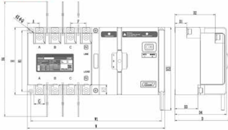
HDQ3S Montaj Boyutları
